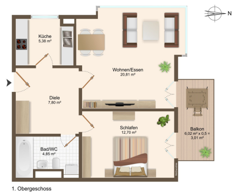
GRUNDRISS!
