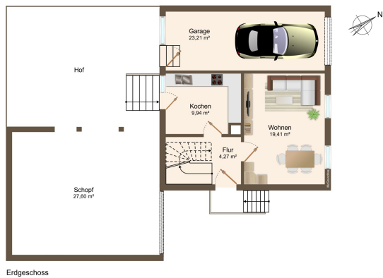
Grundriss Erdgeschoß
