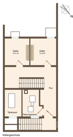
Kellergeschoss
