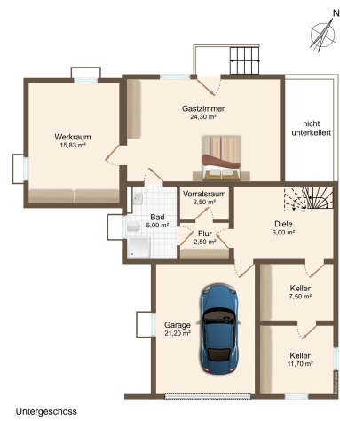
Grundriss Untergeschoß
